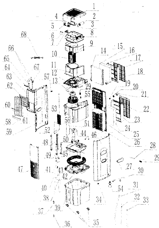
本体分解図
